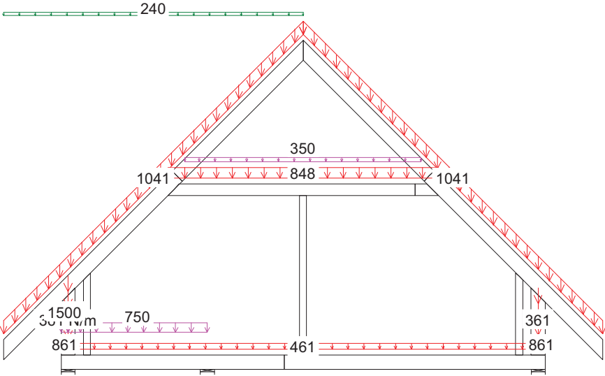
29 Śr Stałe + 0.5*ŚniegL(OP) + OZ2 inne poł. + 0.7*(OZ1 + OZ3), Winst
