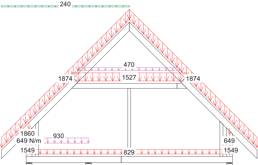
30 Śr 1.8*Stałe + 0.5*ŚniegL(OP)+1.24*OZ2innepoł.+0.94*(OZ1+OZ3), Wfin
