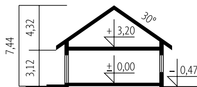
Schemat przekroju
