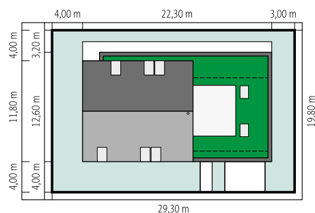
Usytuowanie na działce
