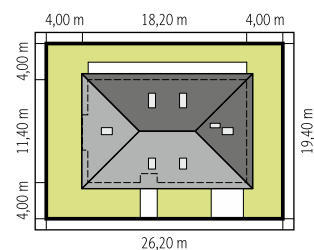
Usytuowanie na działce
