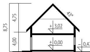
Schemat przekroju
