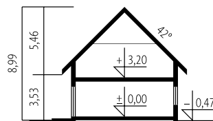
Schemat przekroju
