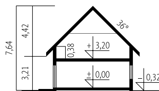
Schemat przekroju
